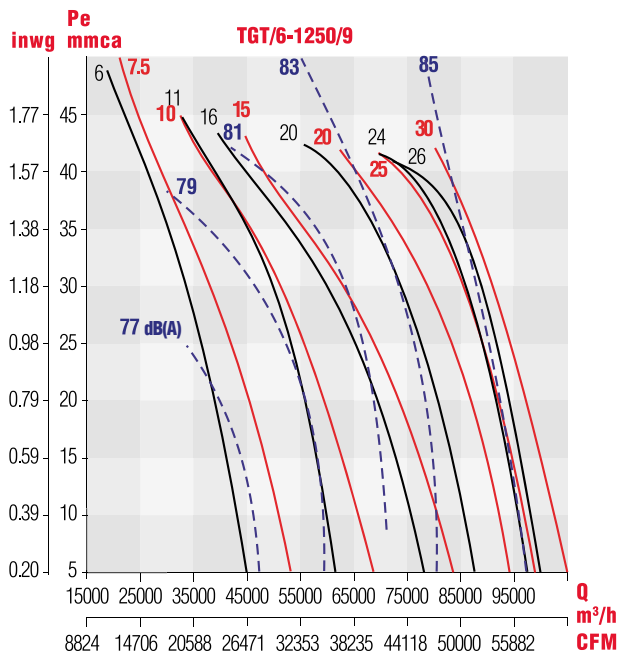
GRÁFICA 11
