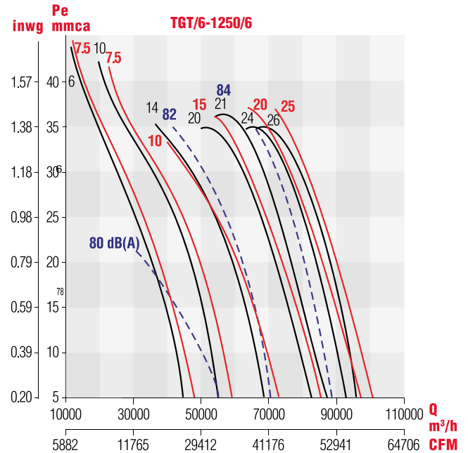
GRÁFICA 10
