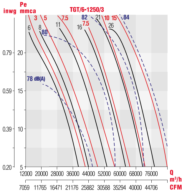
GRÁFICA 9
